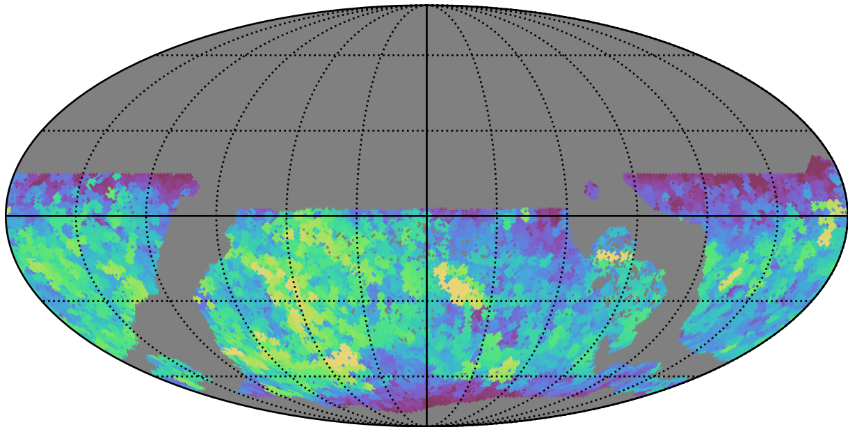
weather_cloudso0v3.4_10yrs WFD z band: Max saturation_mag
