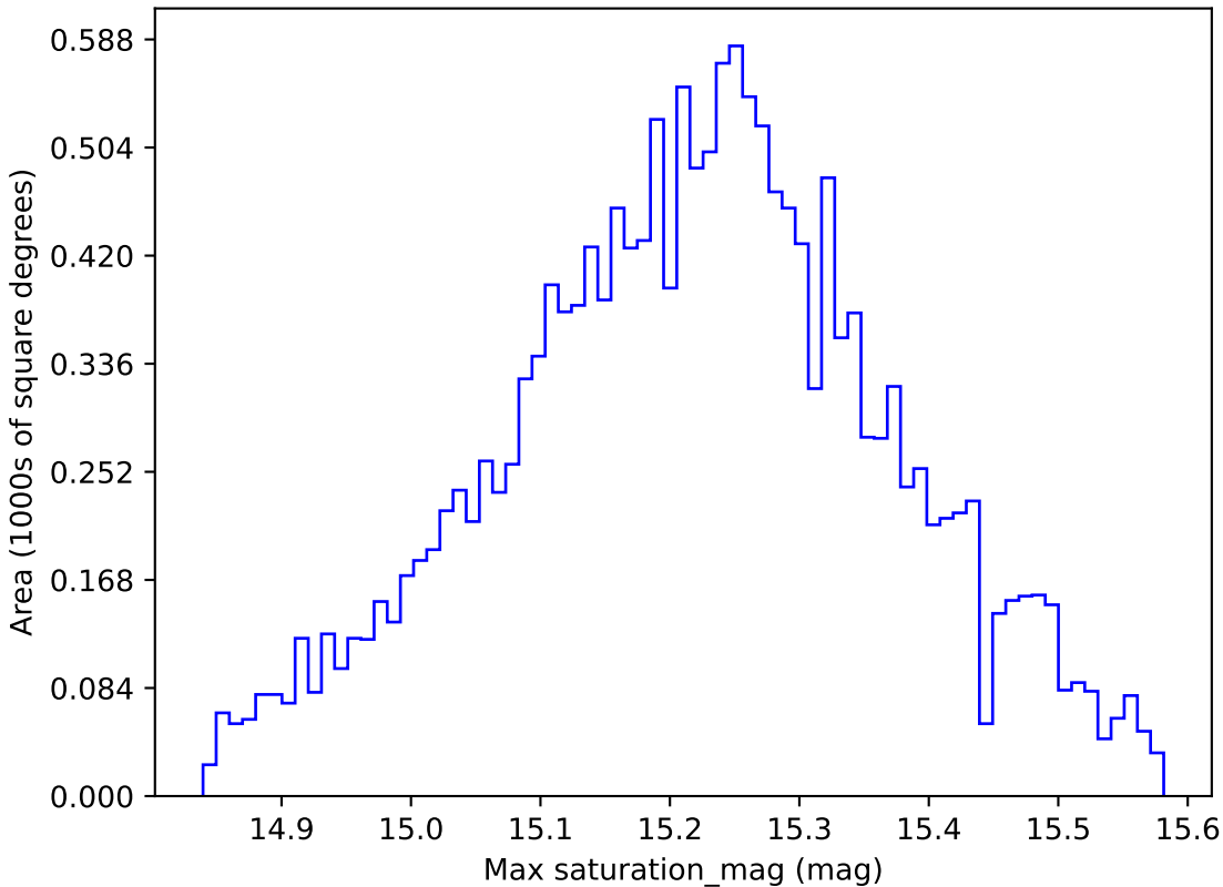
weather_cloudso0v3.4_10yrs WFD z band: Max saturation_mag
