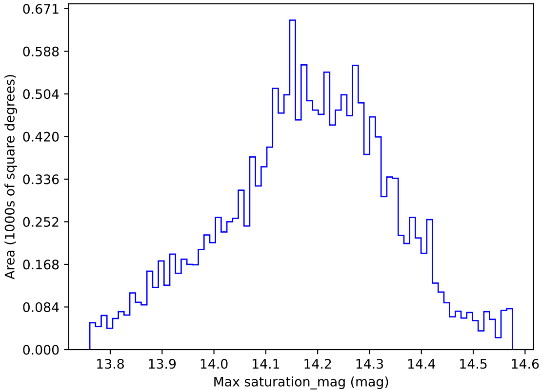
weather_cloudso0v3.4_10yrs WFD y band: Max saturation_mag
