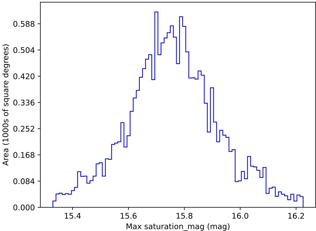
weather_cloudso0v3.4_10yrs WFD r band: Max saturation_mag
