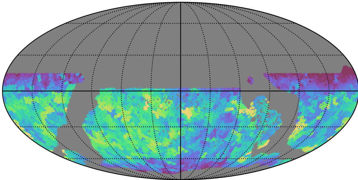
weather_cloudso0v3.4_10yrs WFD i band: Max saturation_mag
