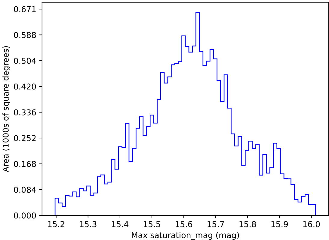
weather_cloudso0v3.4_10yrs WFD i band: Max saturation_mag
