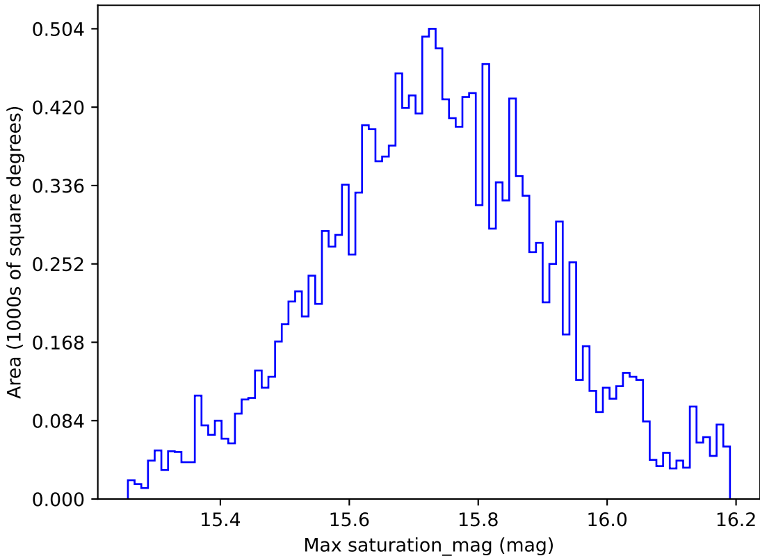
weather_cloudso0v3.4_10yrs WFD g band: Max saturation_mag
