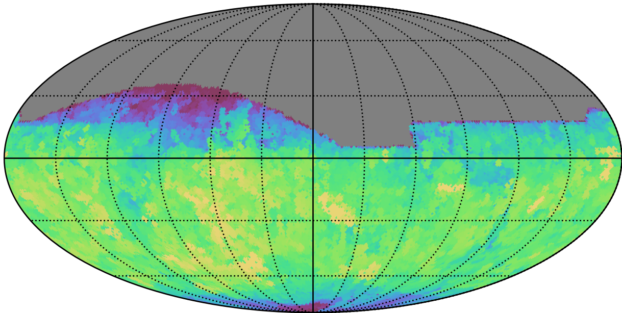
weather_cloudso0v3.4_10yrs All sky z band: Max saturation_mag
