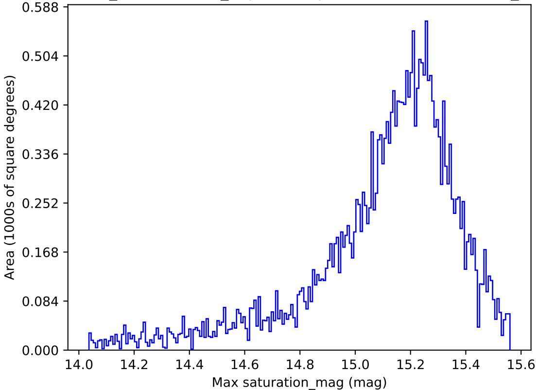
weather_cloudso0v3.4_10yrs All sky z band: Max saturation_mag
