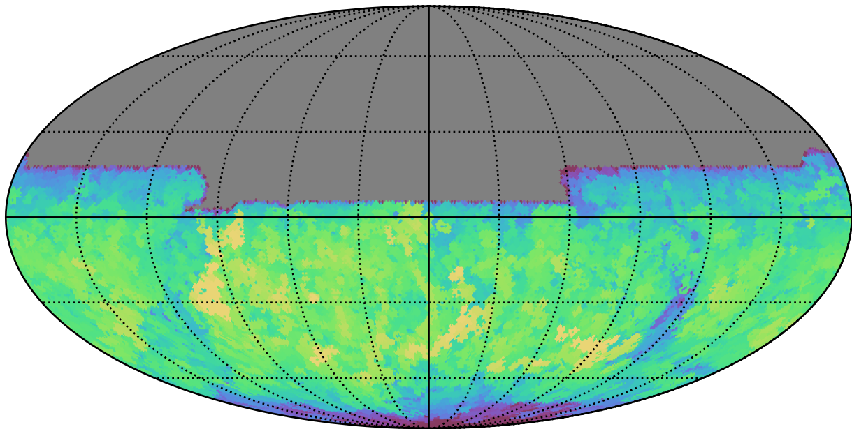
weather_cloudso0v3.4_10yrs All sky y band: Max saturation_mag
