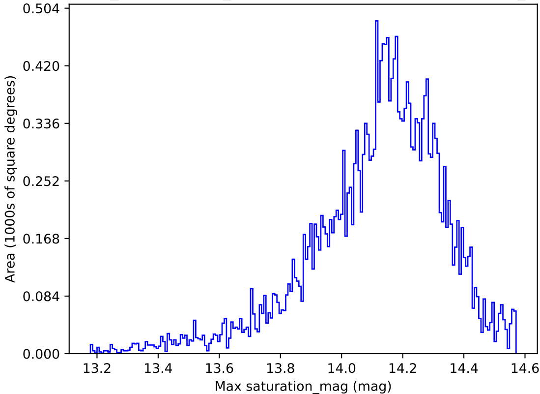
weather_cloudso0v3.4_10yrs All sky y band: Max saturation_mag
