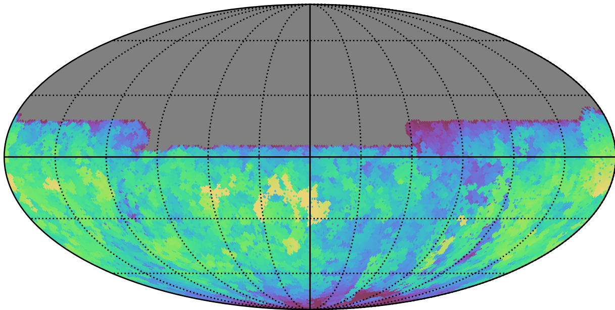
weather_cloudso0v3.4_10yrs All sky u band: Max saturation_mag
