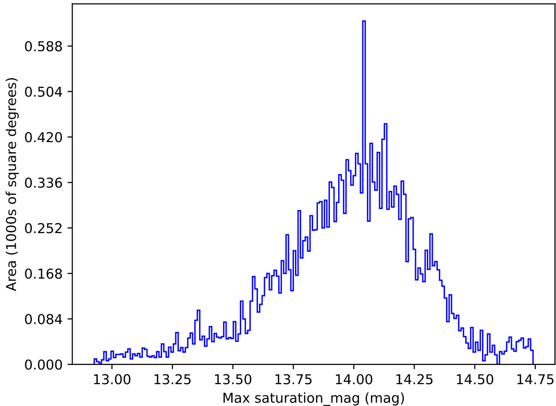
weather_cloudso0v3.4_10yrs All sky u band: Max saturation_mag
