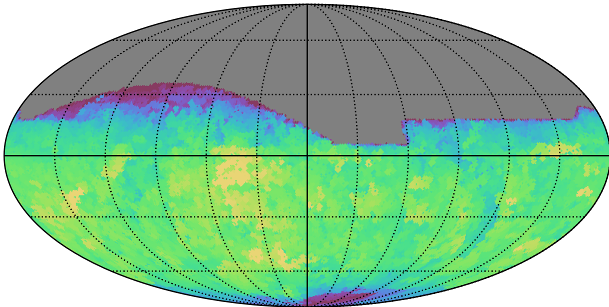
weather_cloudso0v3.4_10yrs All sky r band: Max saturation_mag
