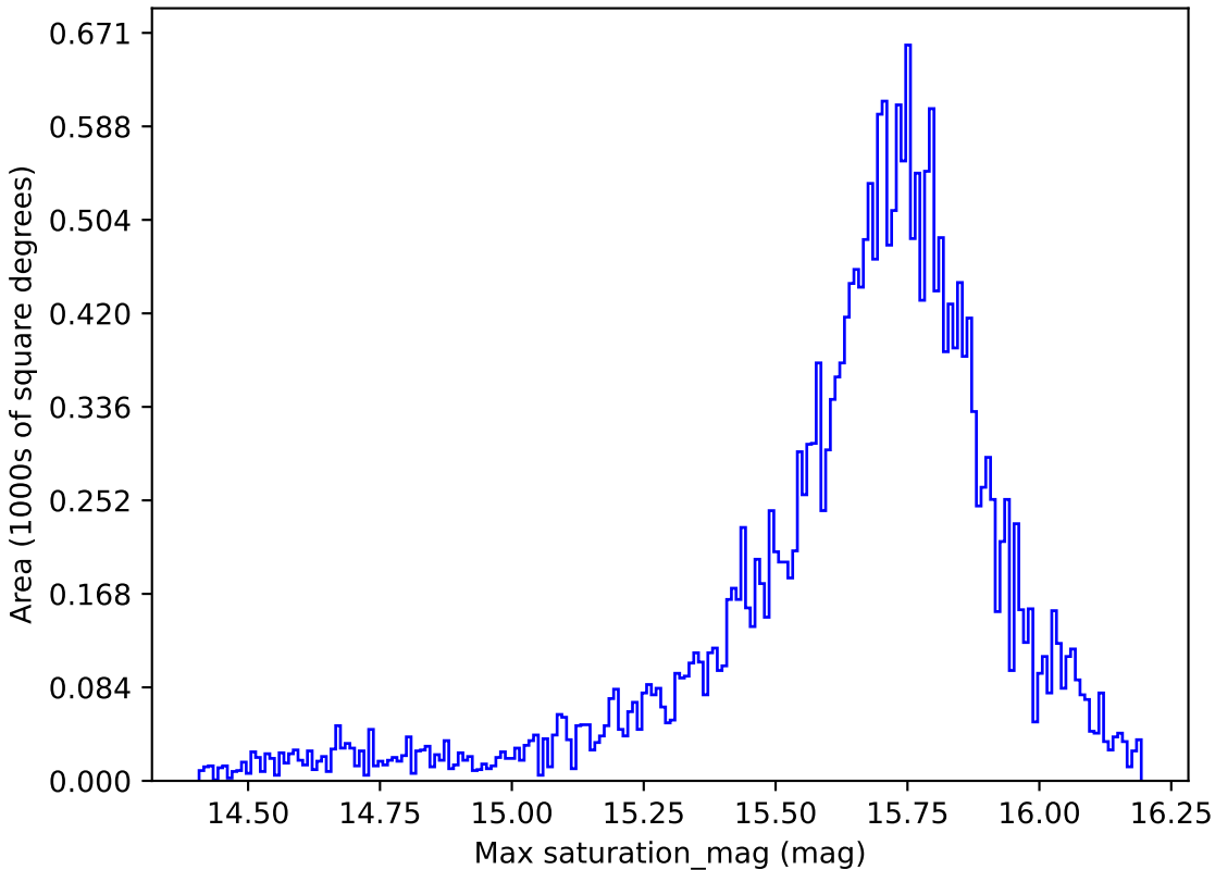
weather_cloudso0v3.4_10yrs All sky r band: Max saturation_mag
