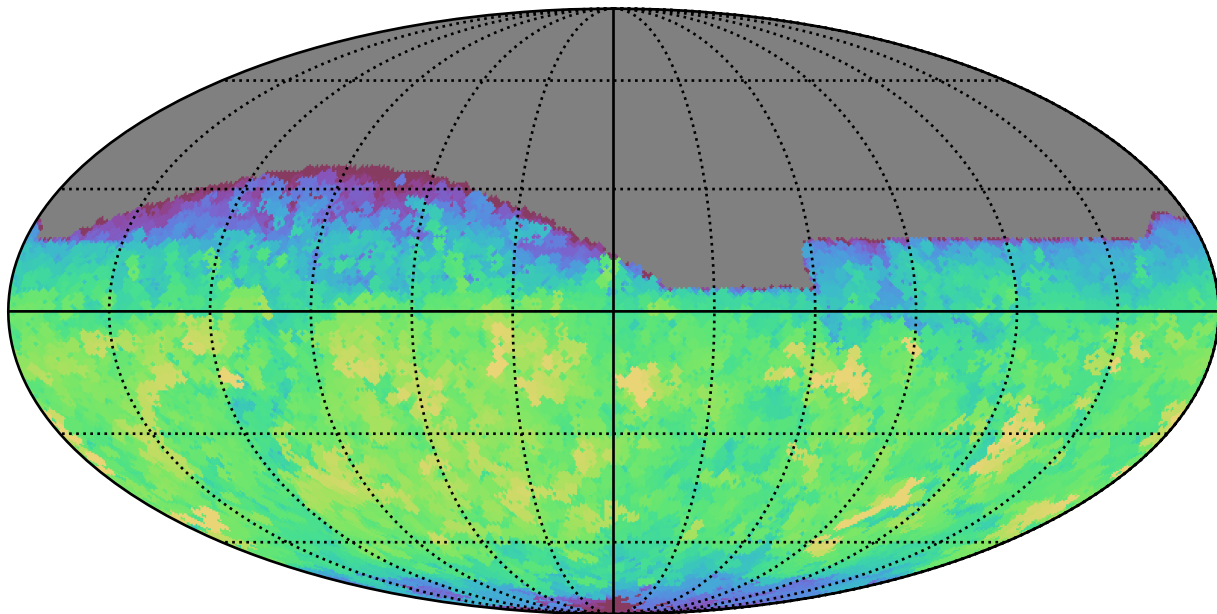
weather_cloudso0v3.4_10yrs All sky i band: Max saturation_mag
