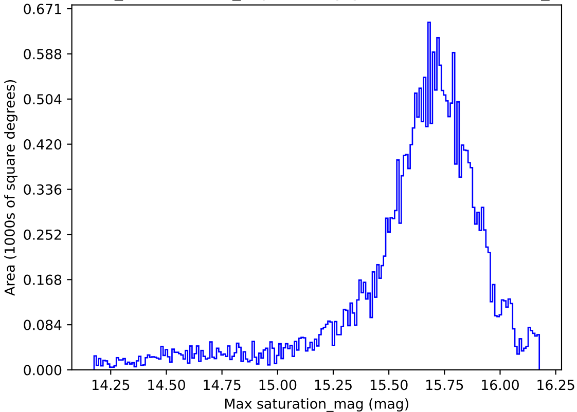
weather_cloudso0v3.4_10yrs All sky g band: Max saturation_mag
