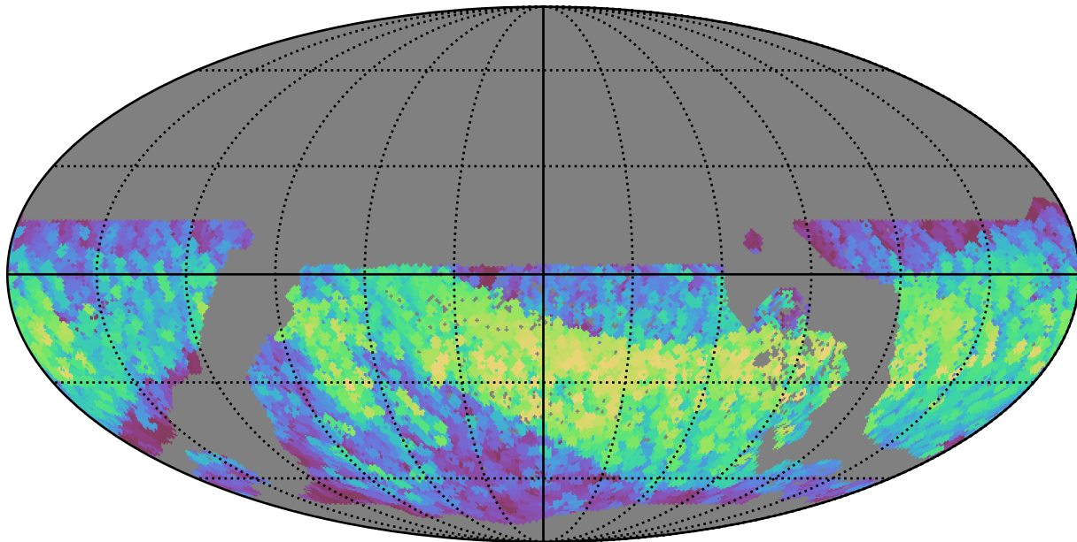
weather_cloudso0v3.4_10yrs WFD z band: Max normairmass
