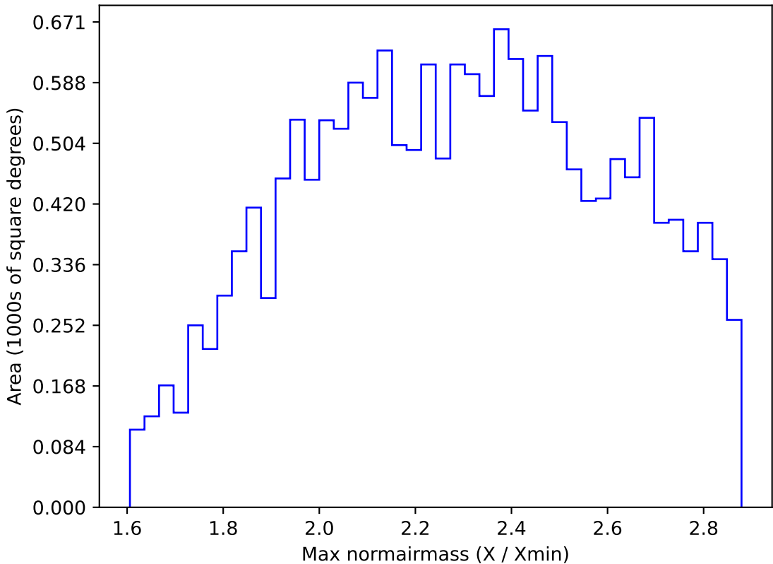
weather_cloudso0v3.4_10yrs WFD z band: Max normairmass
