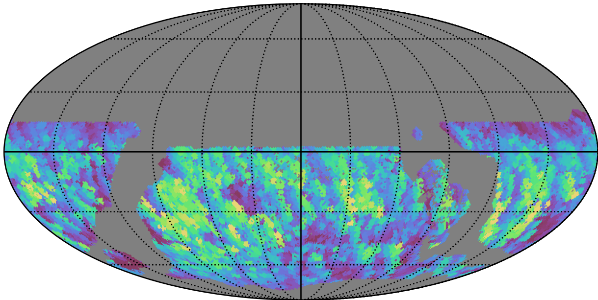
weather_cloudso0v3.4_10yrs WFD y band: Max normairmass
