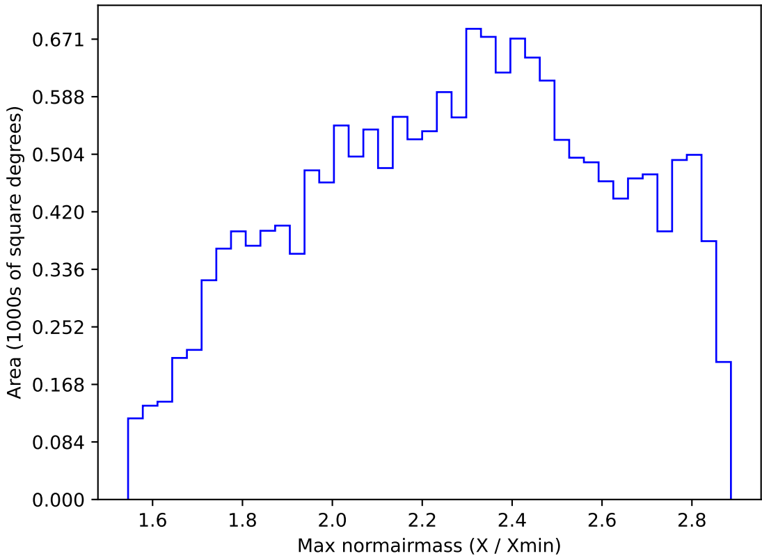
weather_cloudso0v3.4_10yrs WFD i band: Max normairmass
