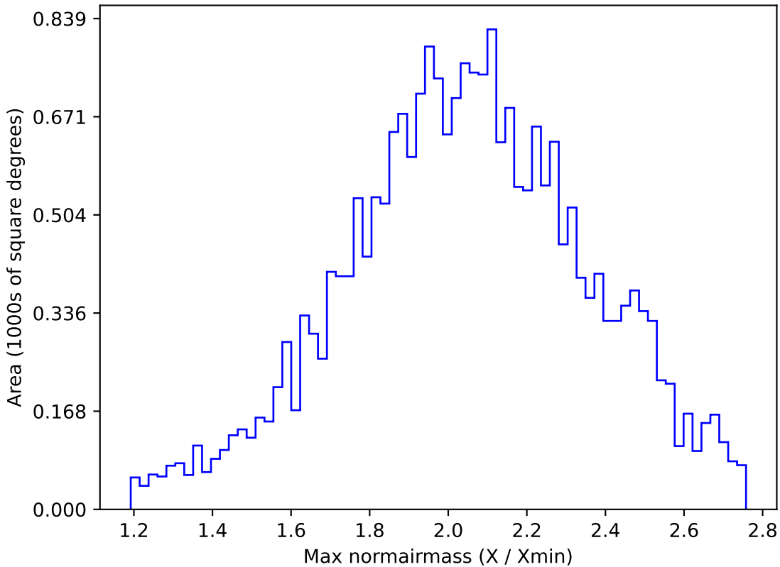
weather_cloudso0v3.4_10yrs All sky y band: Max normairmass
