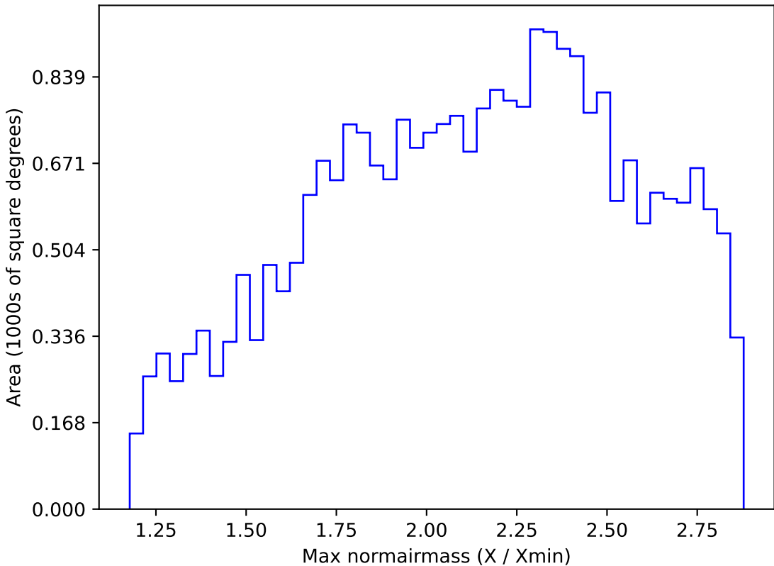
weather_cloudso0v3.4_10yrs All sky i band: Max normairmass
