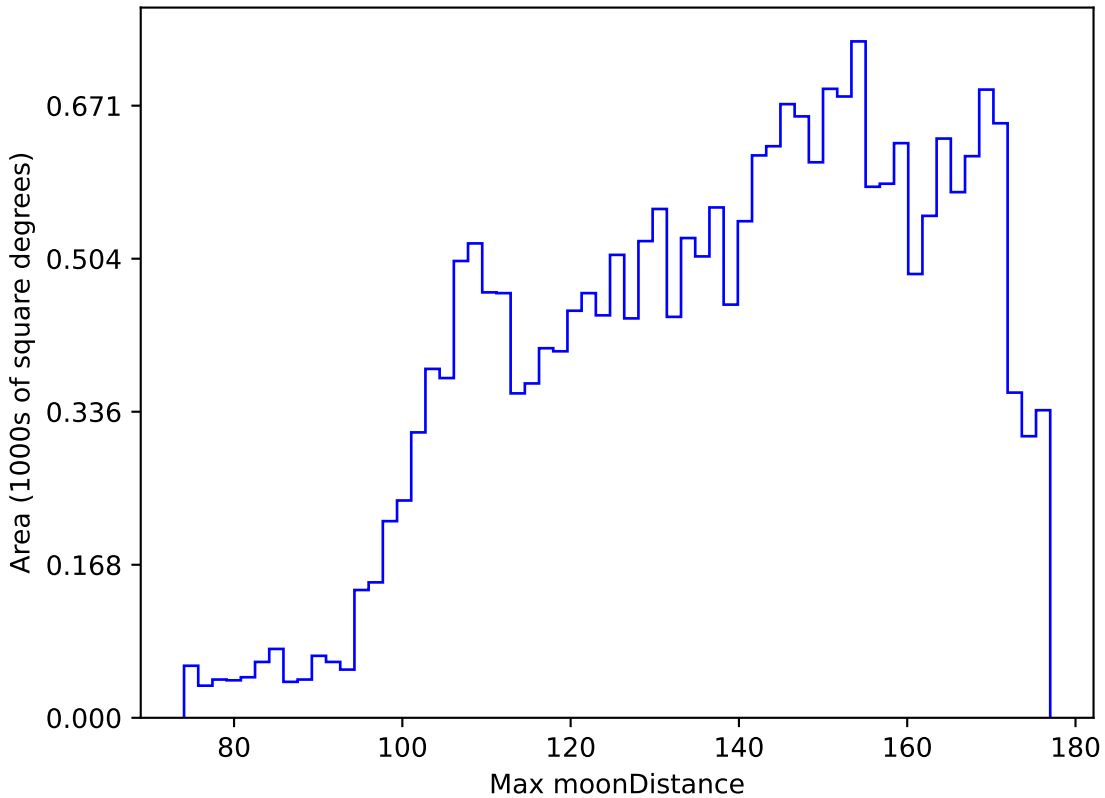
weather_cloudso0v3.4_10yrs All sky y band: Max moonDistance
