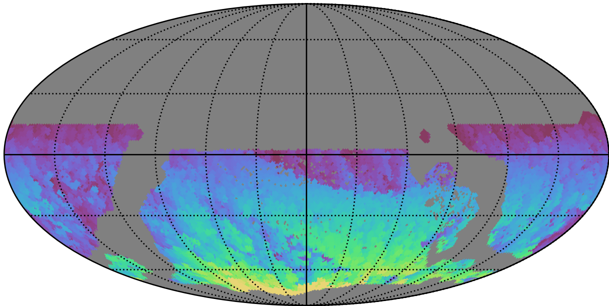
weather_cloudso0v3.4_10yrs WFD z band: Max HA
