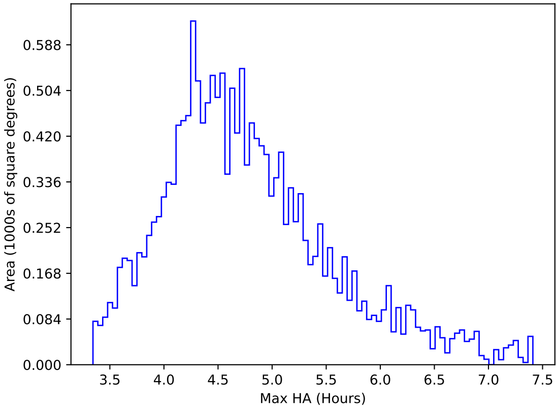
weather_cloudso0v3.4_10yrs WFD y band: Max HA
