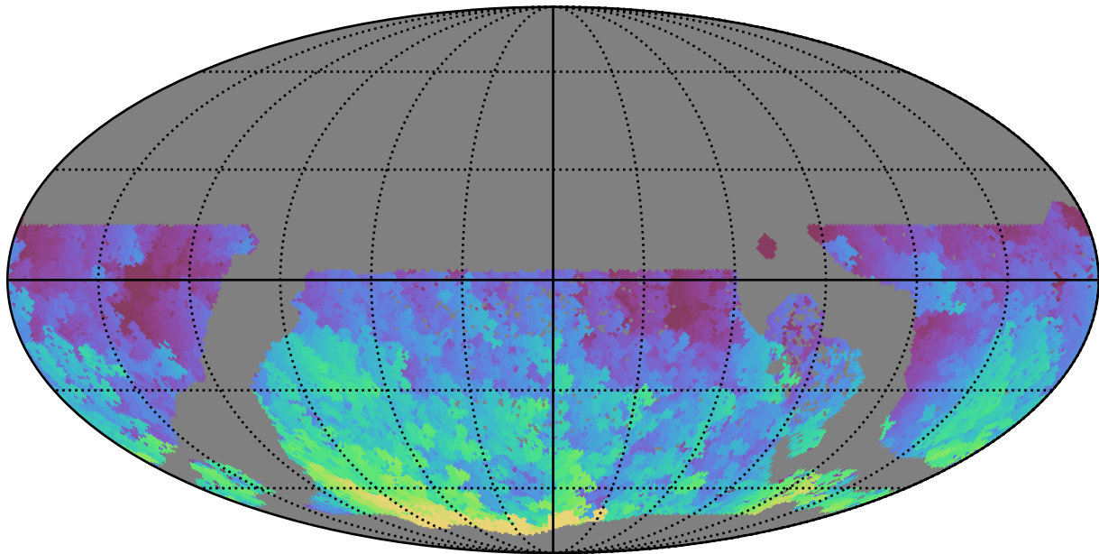
weather_cloudso0v3.4_10yrs WFD u band: Max HA
