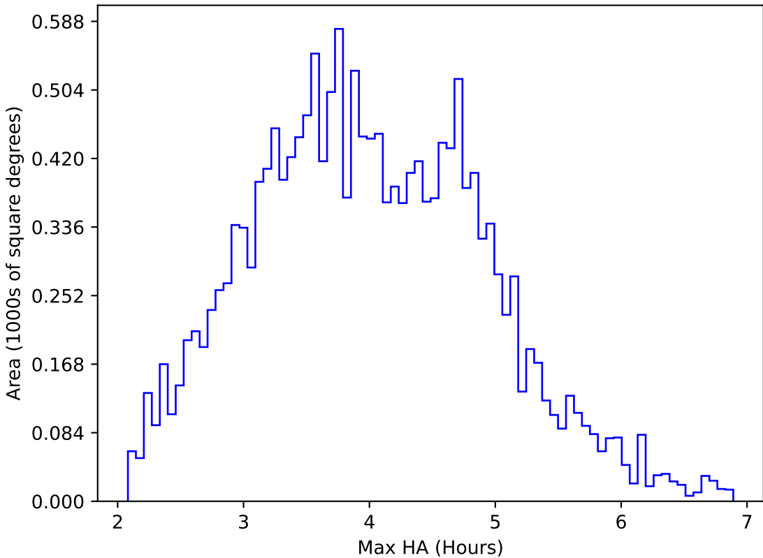
weather_cloudso0v3.4_10yrs WFD u band: Max HA
