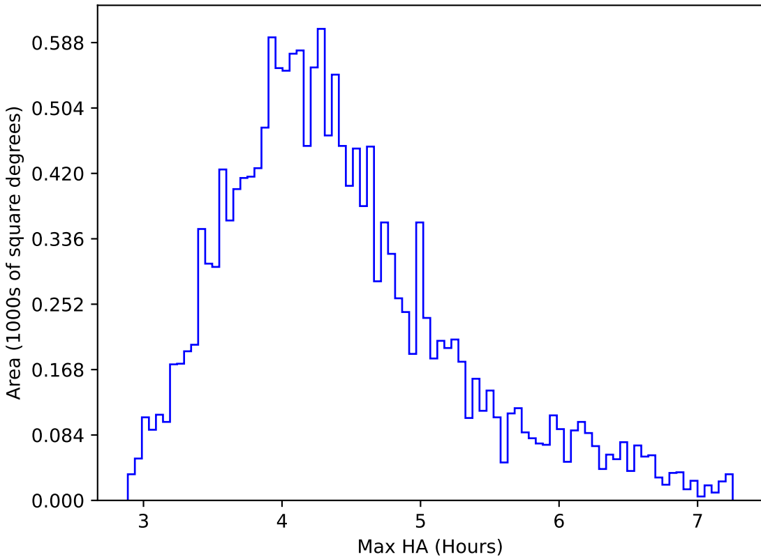
weather_cloudso0v3.4_10yrs WFD r band: Max HA
