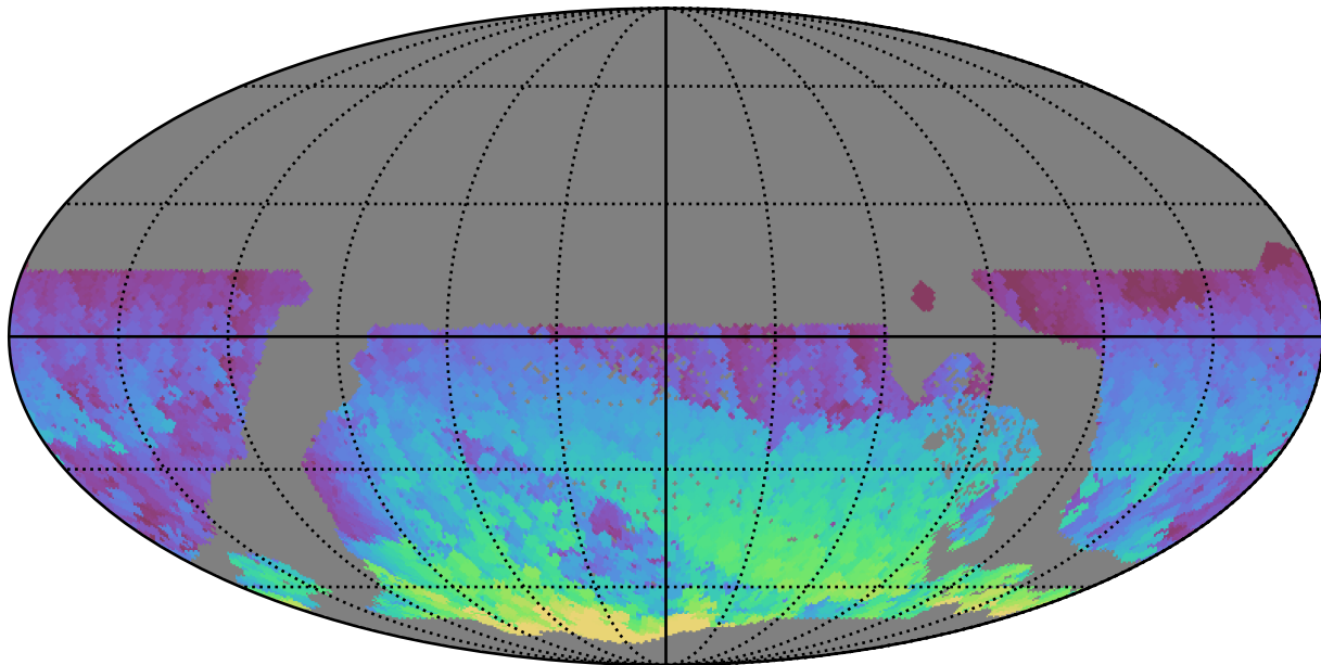
weather_cloudso0v3.4_10yrs WFD i band: Max HA
