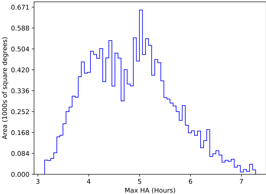
weather_cloudso0v3.4_10yrs WFD i band: Max HA
