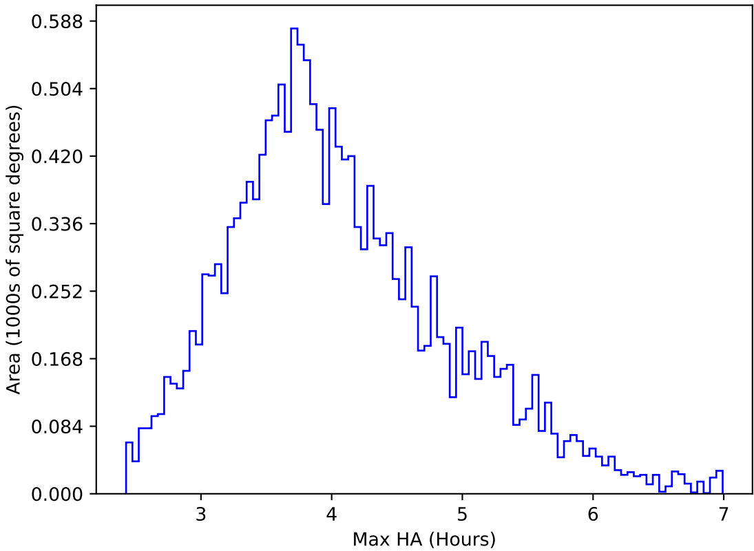
weather_cloudso0v3.4_10yrs WFD g band: Max HA
