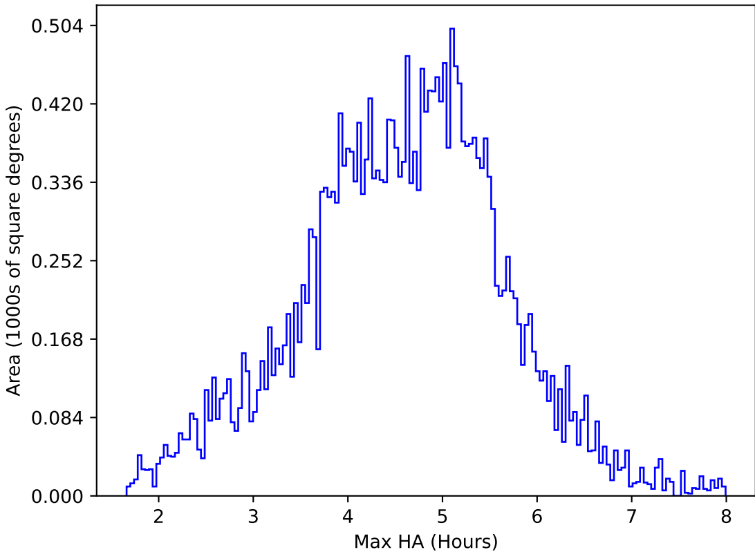
weather_cloudso0v3.4_10yrs All sky z band: Max HA
