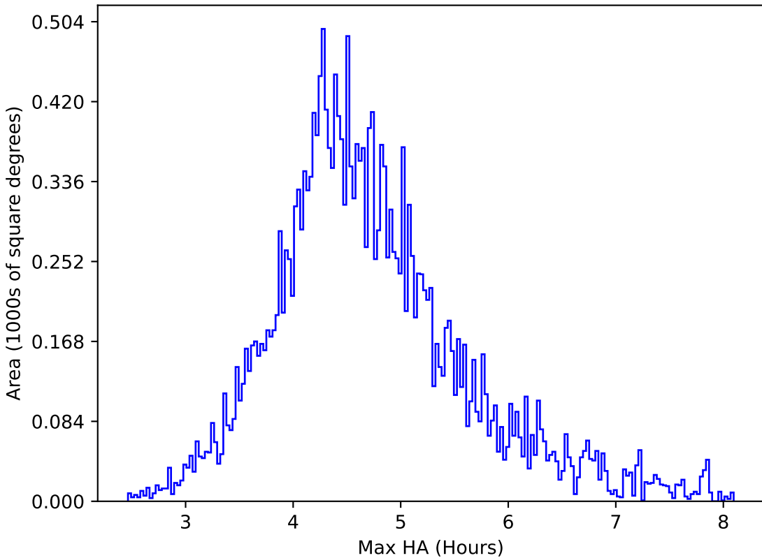
weather_cloudso0v3.4_10yrs All sky y band: Max HA
