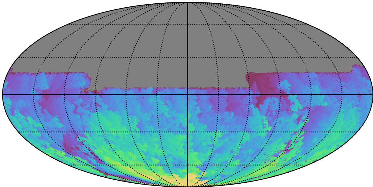
weather_cloudso0v3.4_10yrs All sky u band: Max HA
