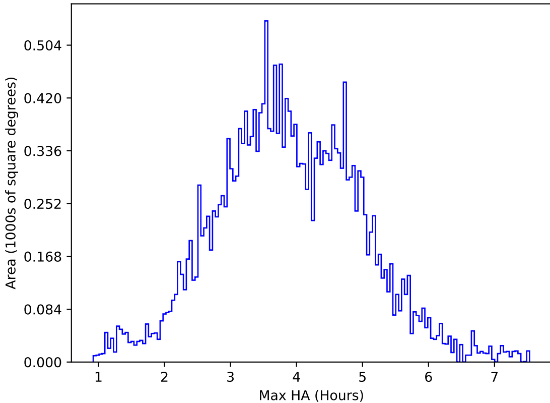
weather_cloudso0v3.4_10yrs All sky u band: Max HA
