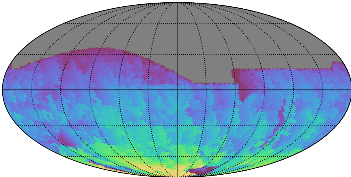
weather_cloudso0v3.4_10yrs All sky r band: Max HA
