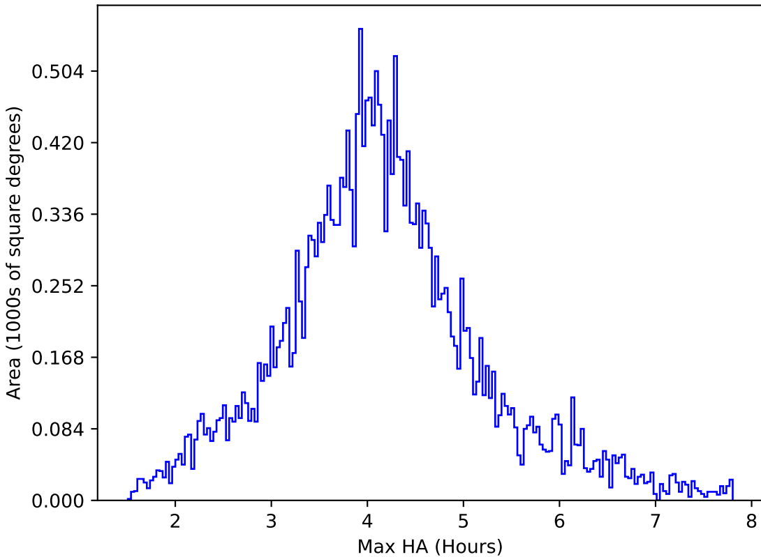
weather_cloudso0v3.4_10yrs All sky r band: Max HA
