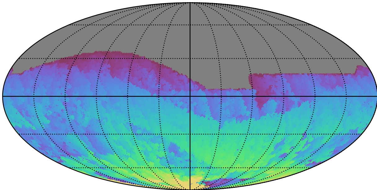
weather_cloudso0v3.4_10yrs All sky i band: Max HA
