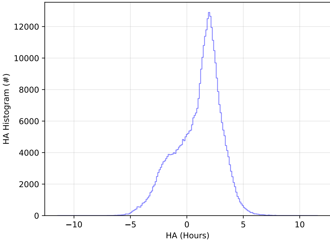
weather_cloudso0v3.4_10yrs WFD y band: HA Histogram
