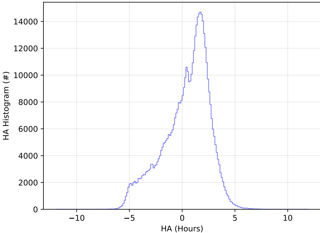
weather_cloudso0v3.4_10yrs WFD r band: HA Histogram
