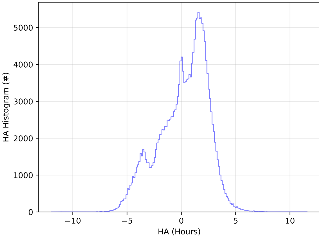
weather_cloudso0v3.4_10yrs WFD g band: HA Histogram
