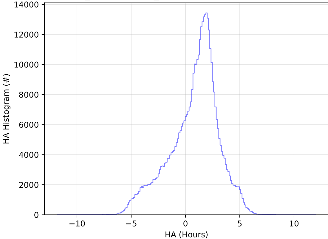
weather_cloudso0v3.4_10yrs All sky z band: HA Histogram
