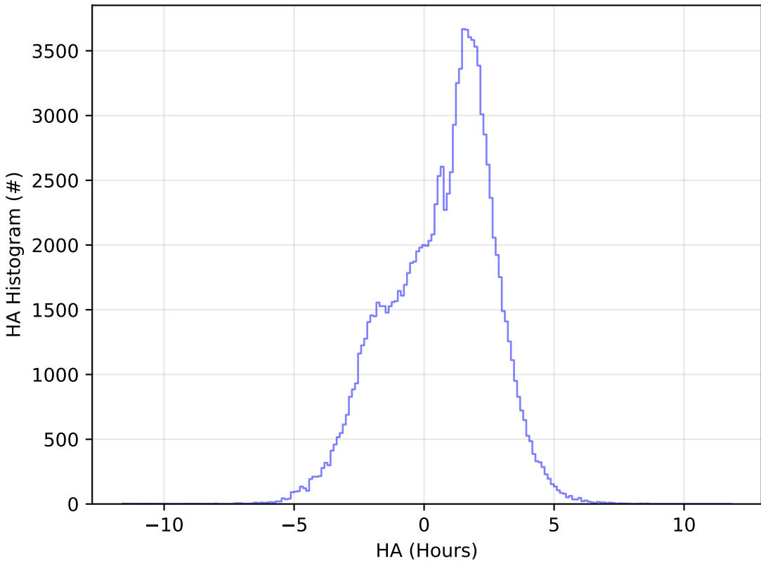
weather_cloudso0v3.4_10yrs All sky u band: HA Histogram
