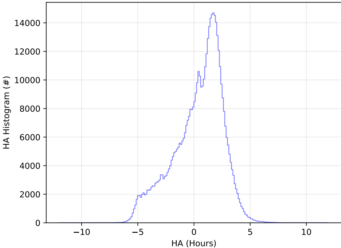
weather_cloudso0v3.4_10yrs All sky r band: HA Histogram
