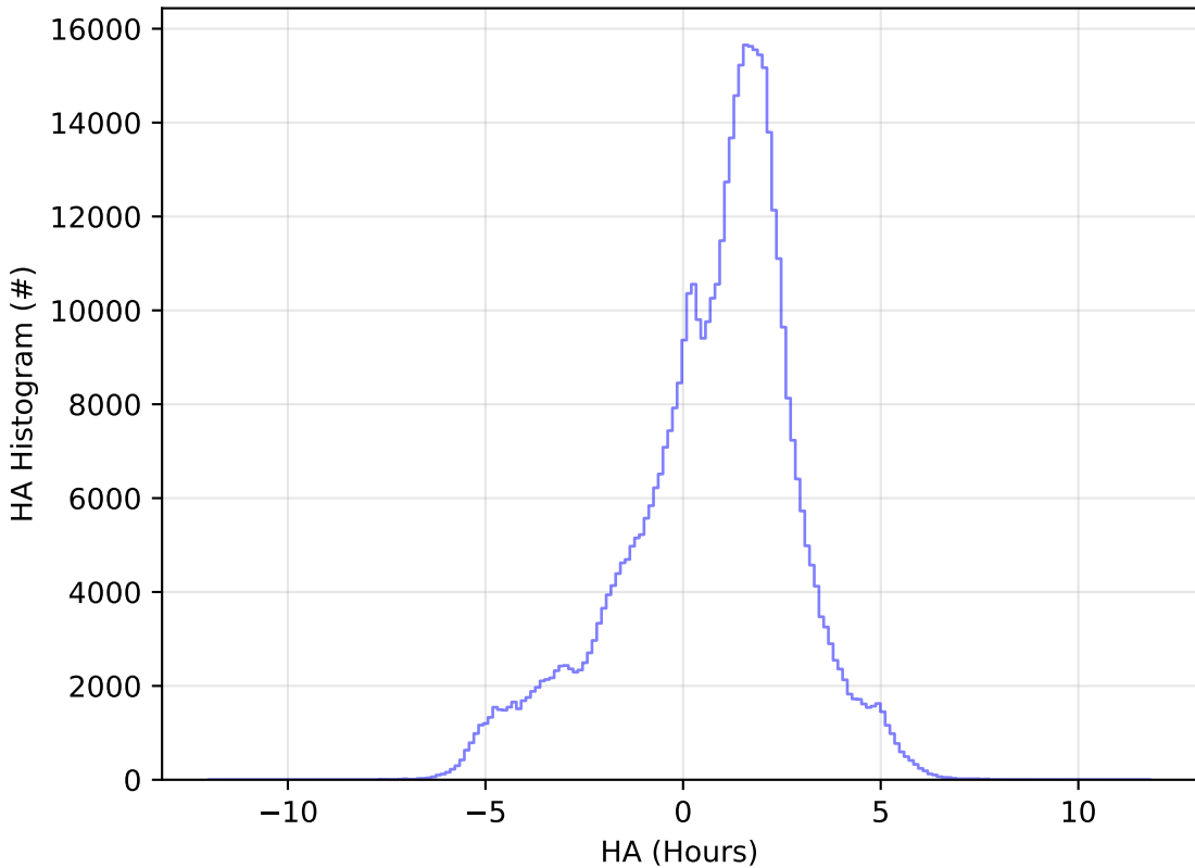
weather_cloudso0v3.4_10yrs All sky i band: HA Histogram
