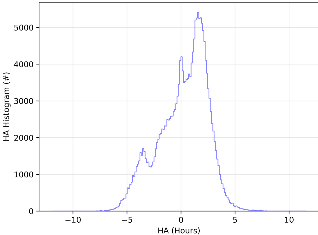
weather_cloudso0v3.4_10yrs All sky g band: HA Histogram
