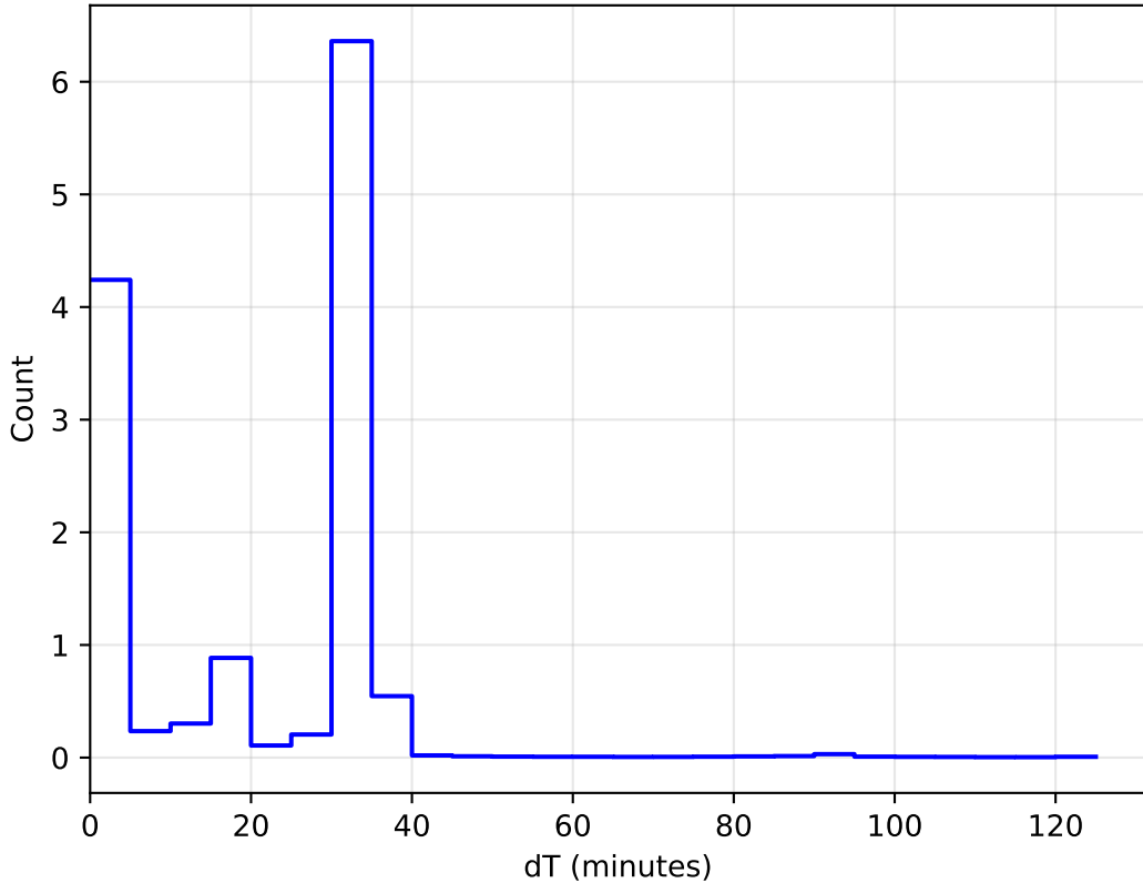
weather_cloudso0v3.4_10yrs All sky: DeltaT Histogram
