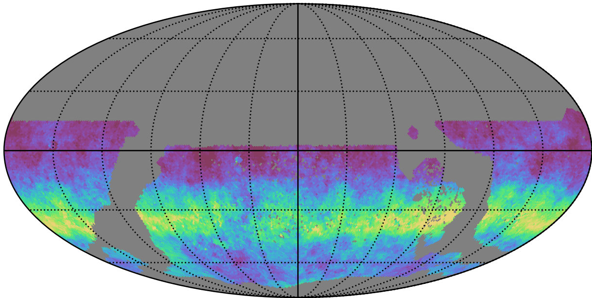
weather_cloudso0v3.4_10yrs WFD g band: AngleRms rotSkyPos
