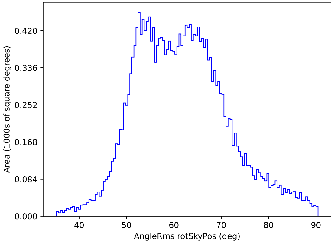
weather_cloudso0v3.4_10yrs All sky y band: AngleRms rotSkyPos
